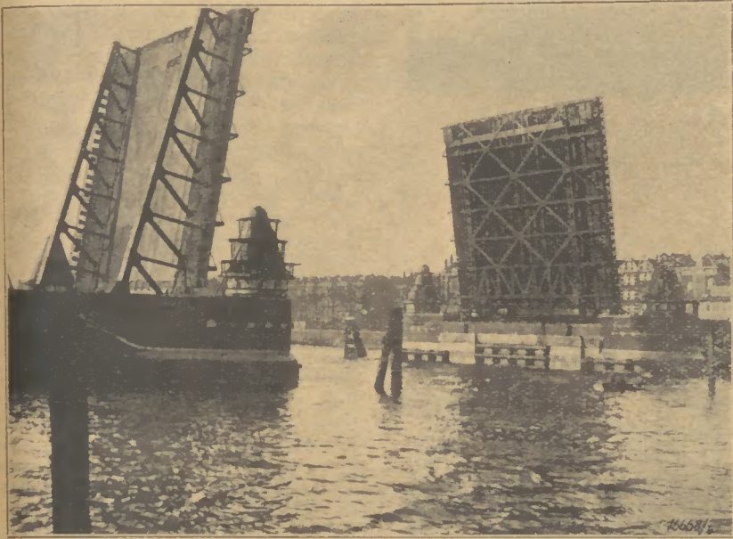
Die neue Königinbrücke in Rotterdam, die gelegentlich des Besuches der Mitglieder des „Vereins Deutscher Ingenieure“ vom Bürgermeister von Rotterdam als Symbol Niederländisch-Deutscher zivilisatorischer Gemeinschaftsarbeit angezogen wurde
