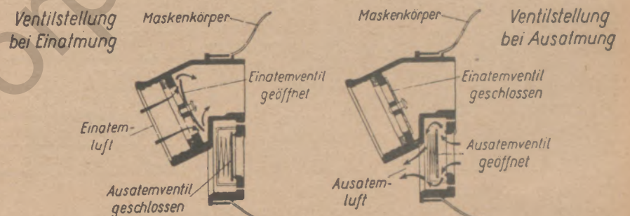
Schnitt durch das Anschlußstück
