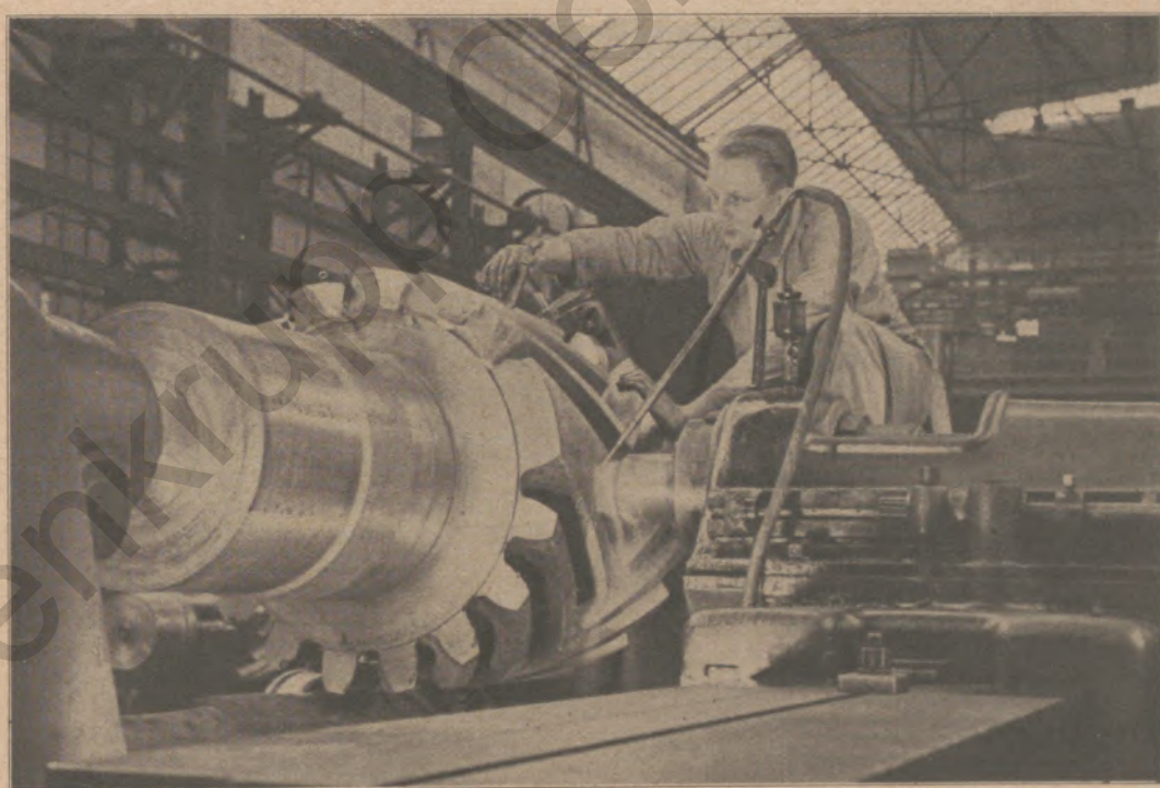
Fräsen von Kammwalzen im Werk Hoerde
