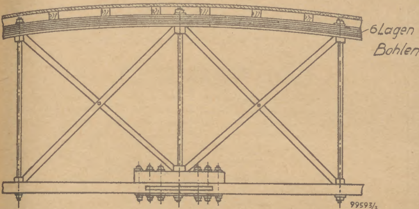
Konstruktion des Stephansbinders
