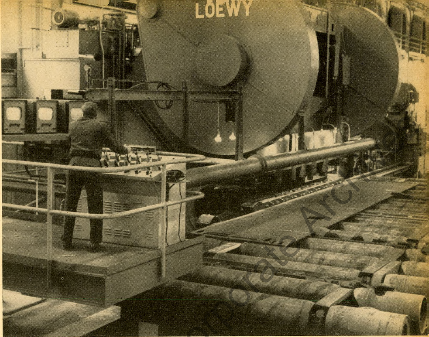
Von seinem Leitstand aus kann der Arbeiter nicht nur über die Fernsehempfänger — die drei Geräte sind links zu erkennen — sämtliche Teile des Glühofens genau kontrollieren, sondern auch die schweren Stahlplatten durch die verschiedenen Stationen der Wärmebehandlungsstraße in der jeweils erforderlichen Geschwindigkeit führen
