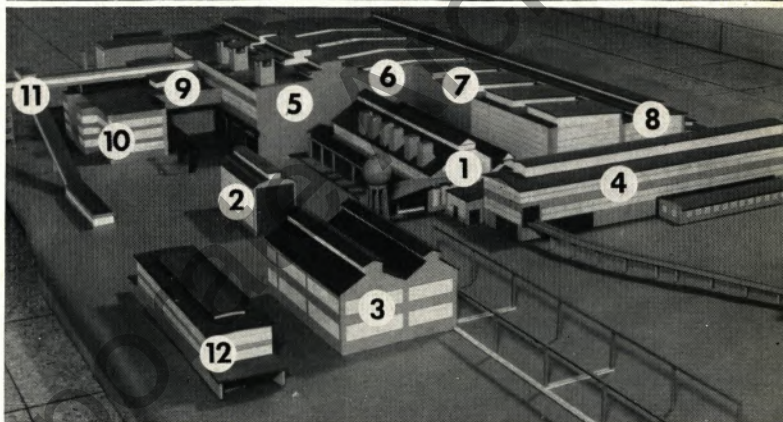
Am Tor 8 in Ruhrort wächst das neue Blasstahlwerk schnell aus dem Boden. Das Gelände hat sich in eine Großbaustelle verwandelt. — Unten: Das Modellfoto zeigt die gesamte Anlage. Die Zahlen bedeuten: 1 vorhandenes Thomaswerk II, 2 Kalkbunker des Thomaswerkes II, 3 Maschinenbetrieb-Werkstatt 9, 4 Elektroofen- und Gießhalle, 5 neue Konverter- und Kaminhalle, 6 Gießhalle, 7 Stripperhalle, 8 Tief-ofenhalle, 9 Dolomit- und Preßwasseranlage, 10 Sozialgebäude für die Belegschaft des neuen Stahlwerkes, 11 Kalktransportbahn, 12 Kalkbunkergebäude
