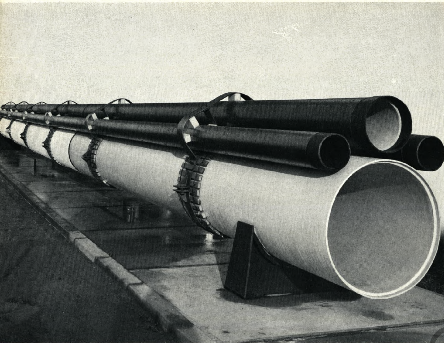
Die Anordnung und Verbindung der vier Rohre, die zusammen das von Laien und Fachleuten vielbeachtete, 320 m lange Dükerbündel durch den Rhein bei Konstanz bilden, sind auf dem Bild deutlich zu sehen. Das große Rohr (NW 800) ist für Abwasser, das darüberliegende Rohr (NW 300) für Trinkwasser vorgesehen. Das Foto zeigt auch die Innenverkleidung der Rohre. Die Hochdruck-Gasleitungen (NW 200) sind seitlich vom Trinkwasserrohr angeordnet.
