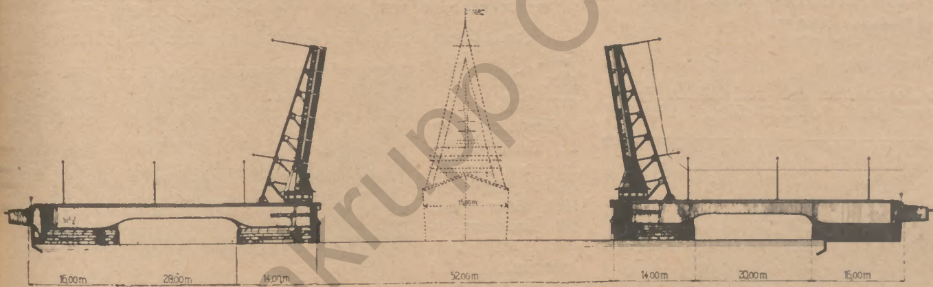
Bild 2: Die Brücke in aufgeklapptem Zustand.
