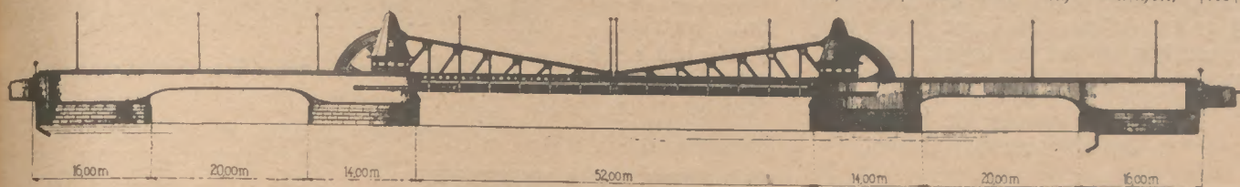
Bild 1: Ansicht der Brücke.
