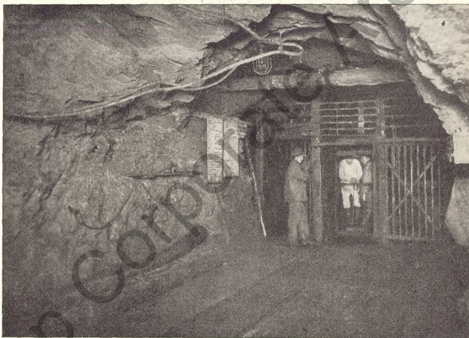
Abb. 9. Steinkohlenwerk Plösch — Füllort auf der 120-m-Sohle
