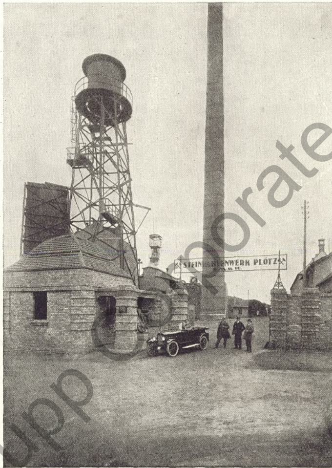
Abb. 2. Steinkohlenwerk Plöb — Zecheneingang
