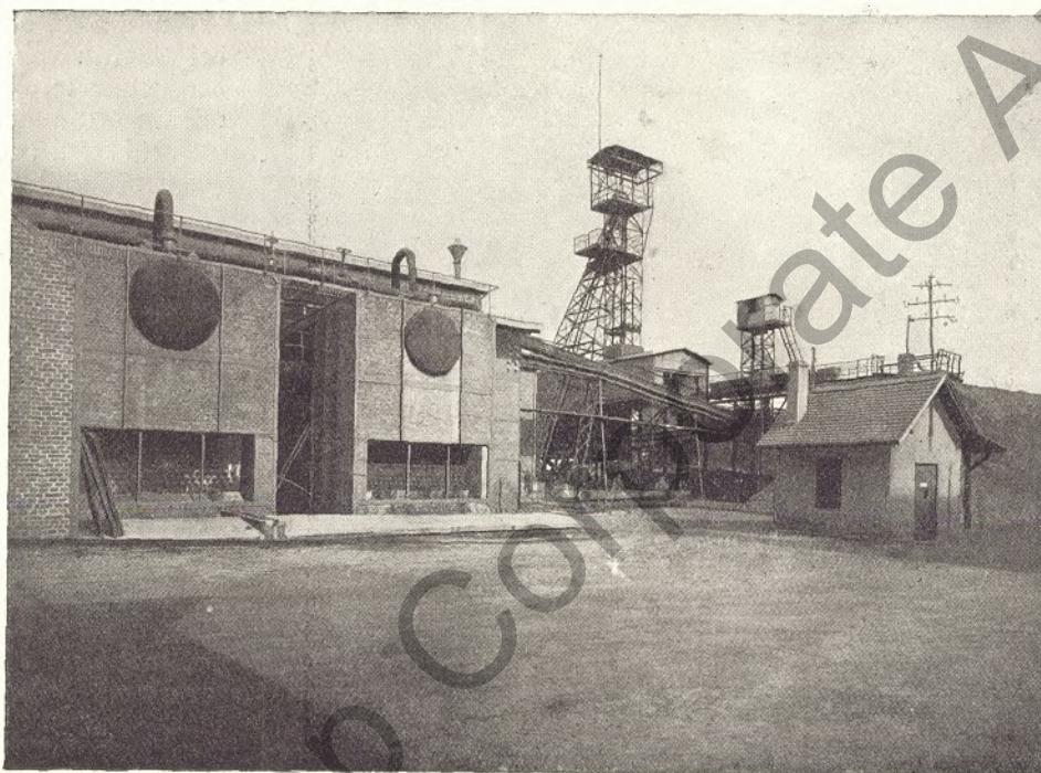
Abb. 3. Steinkohlenwerk Plohn — Kesselhaus und Fördergerüst
