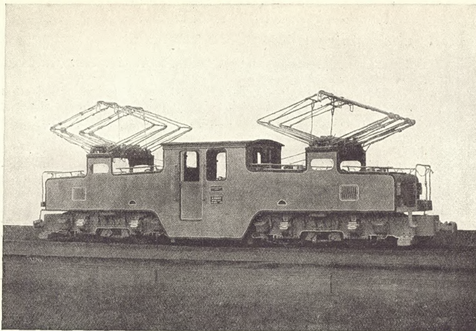
Elektrische Abraumlokomotive von Borsig und Siemens-Schuckert Spurweite 900 mm, Höhe 2,40 m, Gewicht 46 Tonnen, Zugkraft 15 Tonnen
