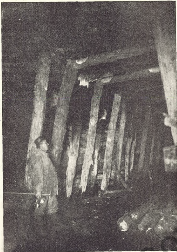
Abb. 10. Steinkohlenwerk Plözh — Strecke im 4 Meter mächtigen Flöz auf der 80-m-Sohle
