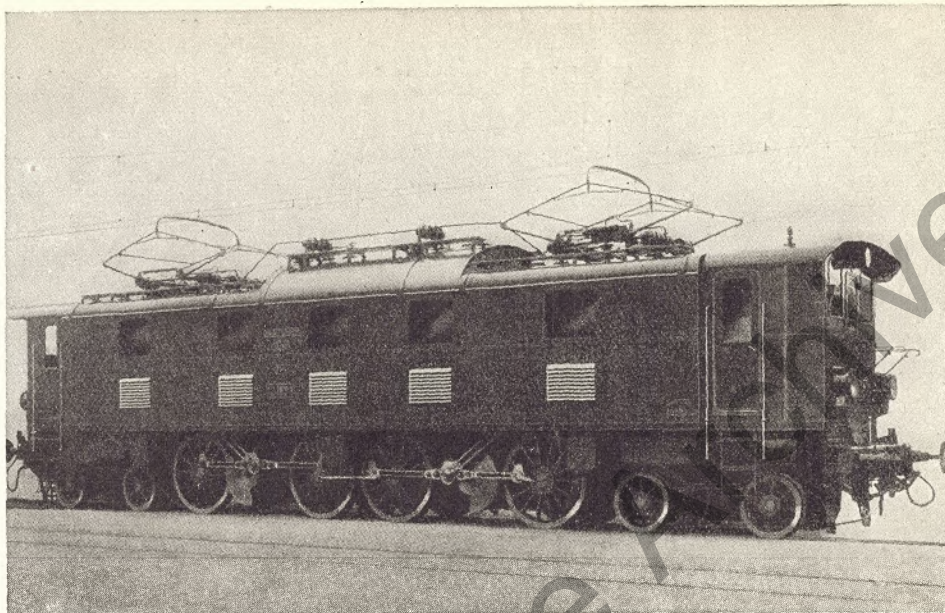
Elektrische 2BB2-Schnellzuglokomotive von Maffei und Siemens-Schuckert Zugfähigkeit 500 Tonnen, 90 km Stundengeschwindigkeit, 17 m lang, 135 Tonnen Gewicht, 15000 Volt Einphasen-Wechselstrom, 4 Motoren zusammen 1440 kW (1960 PS)
