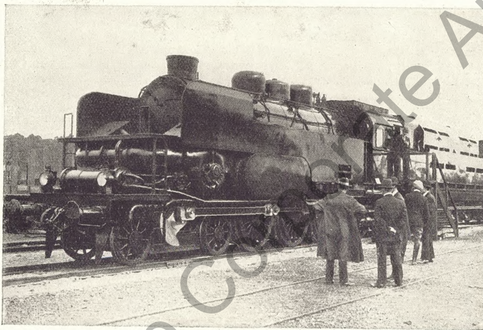
Die Kruppsche Turbinenlokomotive
