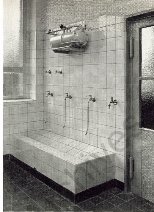
Zur Verhütung von Fußpilz enthalten die Waschräume auch des neuen Belegschaftshauses der Breitbandstraße Spezialreinigungsanlagen, die sich bewährten
