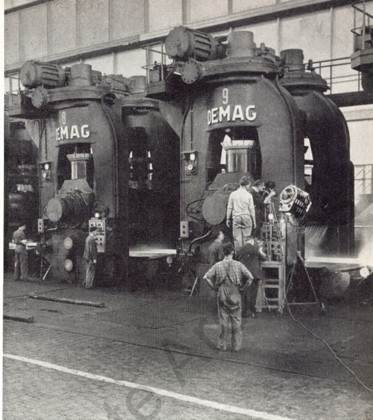
Die Fertigstraße wird bei den Aufnahmen zum Werkfilm mit Scheinwerfern „ausgeleuchtet“. Während der Dreharbeiten konnten die Kameramänner nie nahe genug „herankommen“
