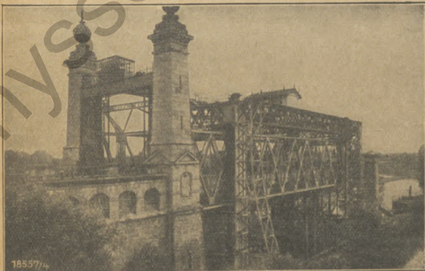
Schiffshebewerk am Dortmund-Ems-Kanal bei Henrichenburg
