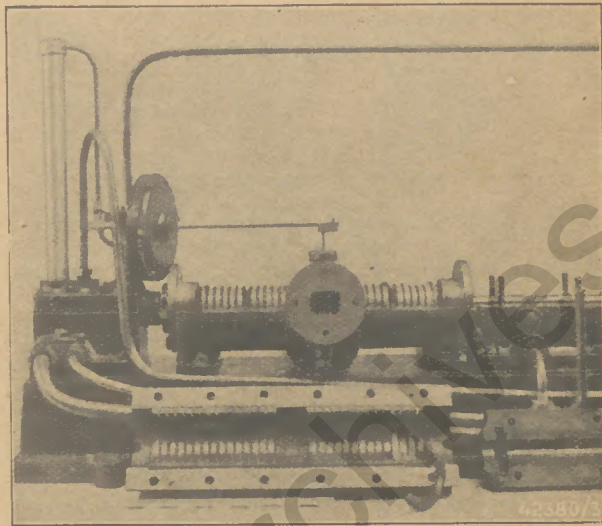
Abb. 2: Turbine von Parsons vom Jahre 1884
