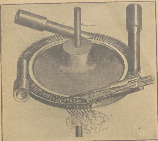
Abb. 1: De Laval's Turbinenrad aus dem Jahre 1883
