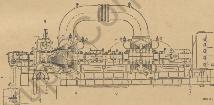
Abb. 3: Turbogenerator für die HEW.; Leistung 35 000 bis 38 500 kW/St.; Umlaufzahl: 3000 in der Minute
