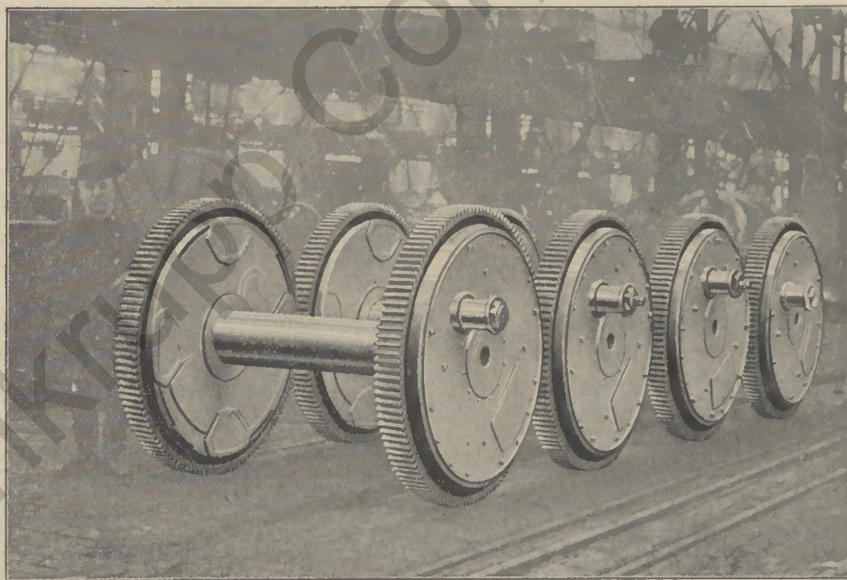
Getriebe für elektrische Lokomotiven der nordwegischen Staatsbahnen
