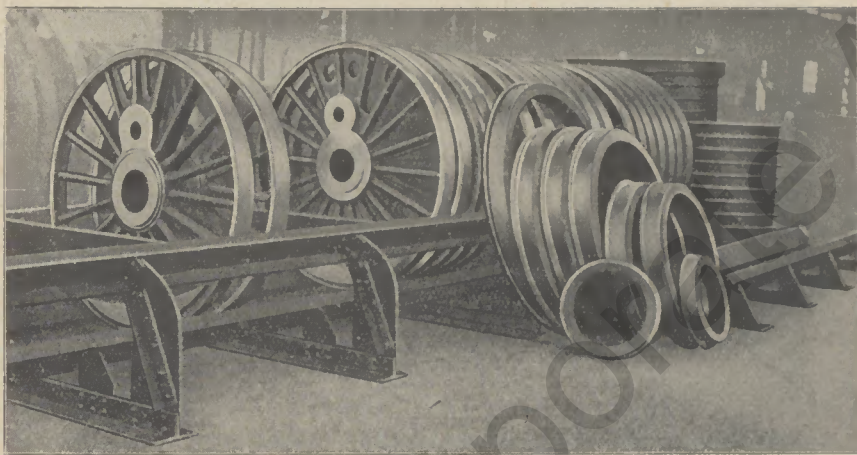
Radsterne und Radreifen für Lokomotiv-, Tender- und Wagenradfäße
