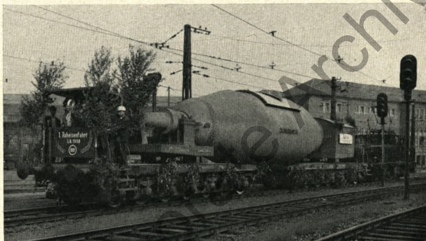
Die neue Roheisen-Torpedo-Pfanne, die Roheisen von den Ruhrorter Hochöfen zum Mischer des Blasstahlwerkes transportiert, hat am 1. Juni 1959 ihre erste Fahrt gemacht (s. Heft 28)
