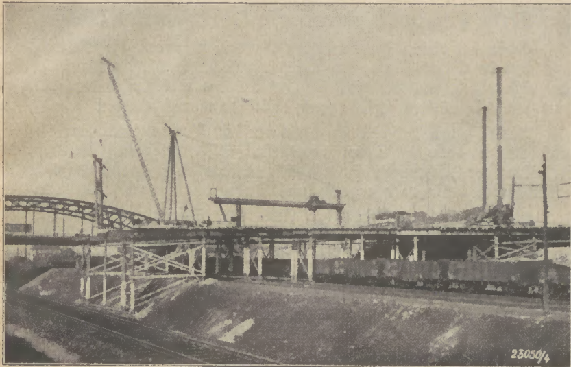
Der Beginn der Montagearbeiten für den Bau der „Schnettkerbrücke“ in Dortmund
