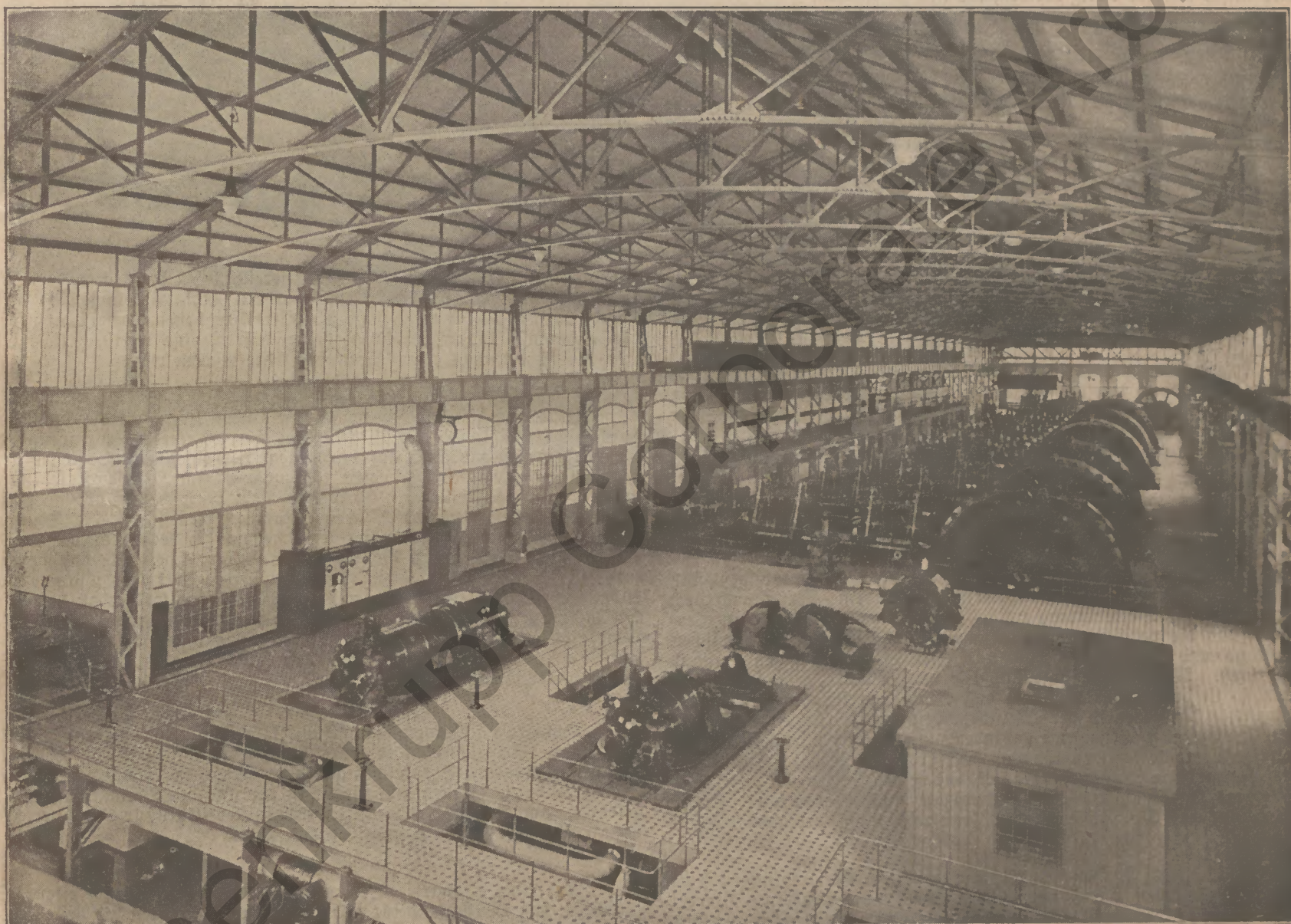
Neuzeitliches Hochofen-Kraftwerk
