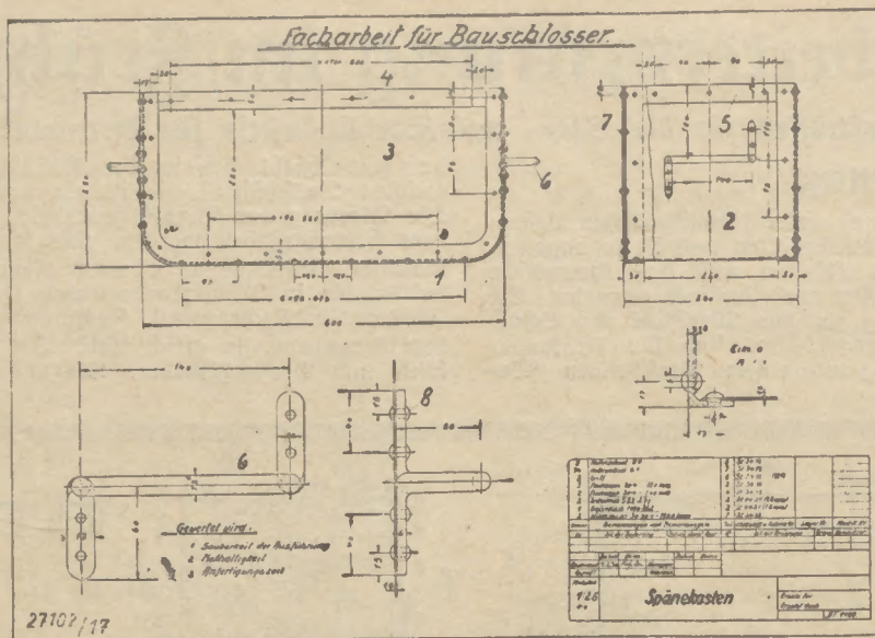
Bild 3. Facharbeit für Bauschlosser: Spänekasten. Aufgabe
