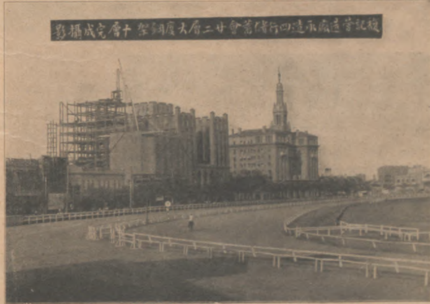
Links: Bild auf Stahlskelett und Schwentreife bei der Montage. — Rechts: Das Hochhaus im Bau; im Vordergrund die Reitbahn; rechts neben dem Hochhaus das Heim des „Vereins christlicher junger Männer U.S.M.“. Das Heim ist hervorragend eingerichtet, besitzt Schwimmbad usw. und nimmt auch Nichtamerikaner auf. Das nächste Haus rechts ist ein großes Warenhaus wie z. B. Althoff in Dortmund.
