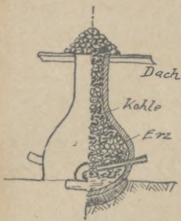
Abb. 1. Schmelzofen in Kamerun, aus 5 bis 6 cm starken Ziegeln erbaut
