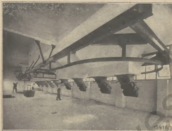
Abb. 10: (links oben) Innenansicht des mittleren Bunker- teiles, Transport- schnecken mit Schalt- anlage
