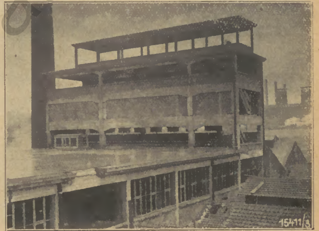
Abb. 4: Südwestliche Ansicht des im Rohbau fertigen Bunkerbaues. Bauzustand am 23. 2. 28
