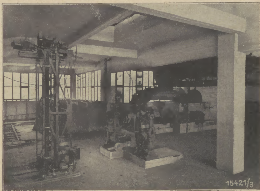
Abb. 14: Strangpresse
