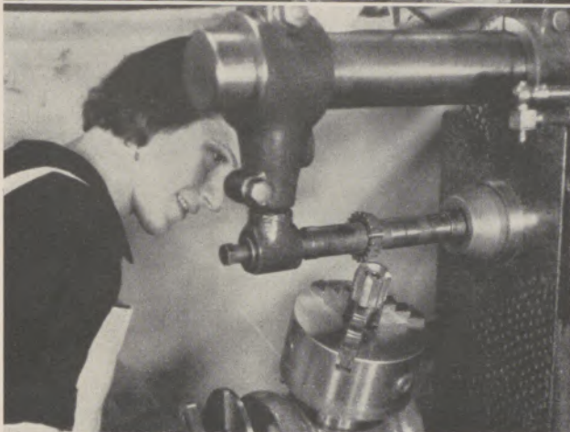
Bild 3: Einsetzen der Schneiden in einen Formfräser (oben links)
