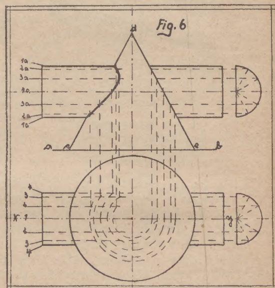
Kegel von einem Zylinder durchdrungen.
