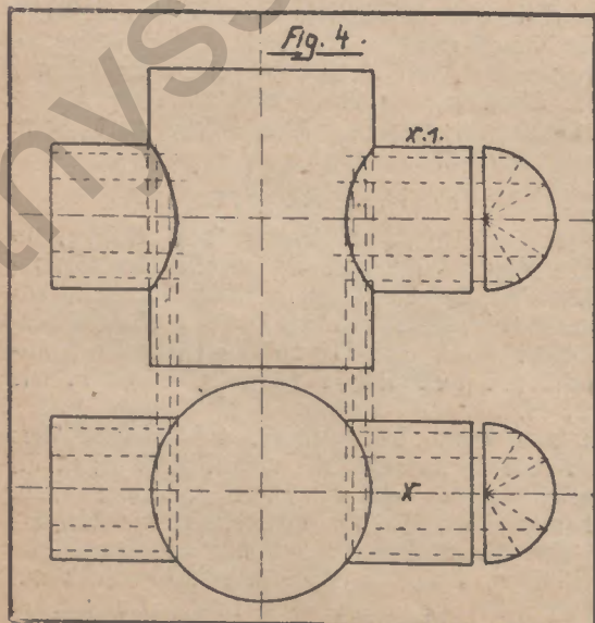
Größerer Kreiszylinder von einem kleineren Kreiszylinder rechtwinklig durchdrungen.
