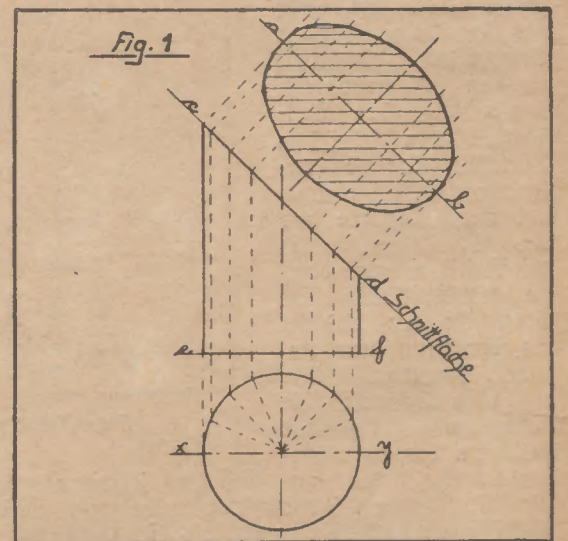
Schräg durch die Achse geschnittener Zylinder.
