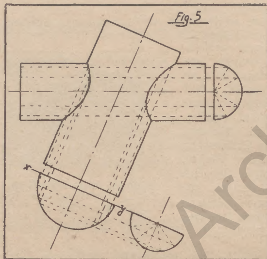
Größerer, geneigt liegender Zylinder von einem kleineren Zylinder schiefwinklig durchdrungen.
