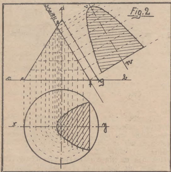
Kegelschnitt schräg durch die Achse, parallel einer Erzeugungsline.
