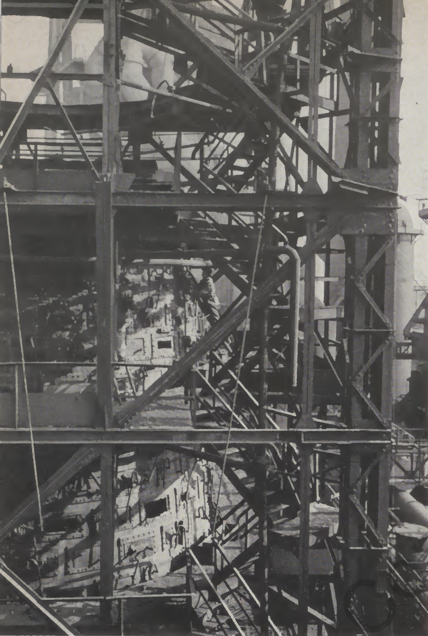
Demontage 1960: Kaum noch als Hochofen identifizierbar ist das Stahlgerüst, das noch immer den Ofenschacht umschließt; (o.); doch schon rücken die Schneidbrenner auch dem Panzer zu Leibe (u.). Bei der Demontage eines Winderhitzers (o. r.) erkennt man den aus 60 000 Gittersteinen bestehenden Besatz
