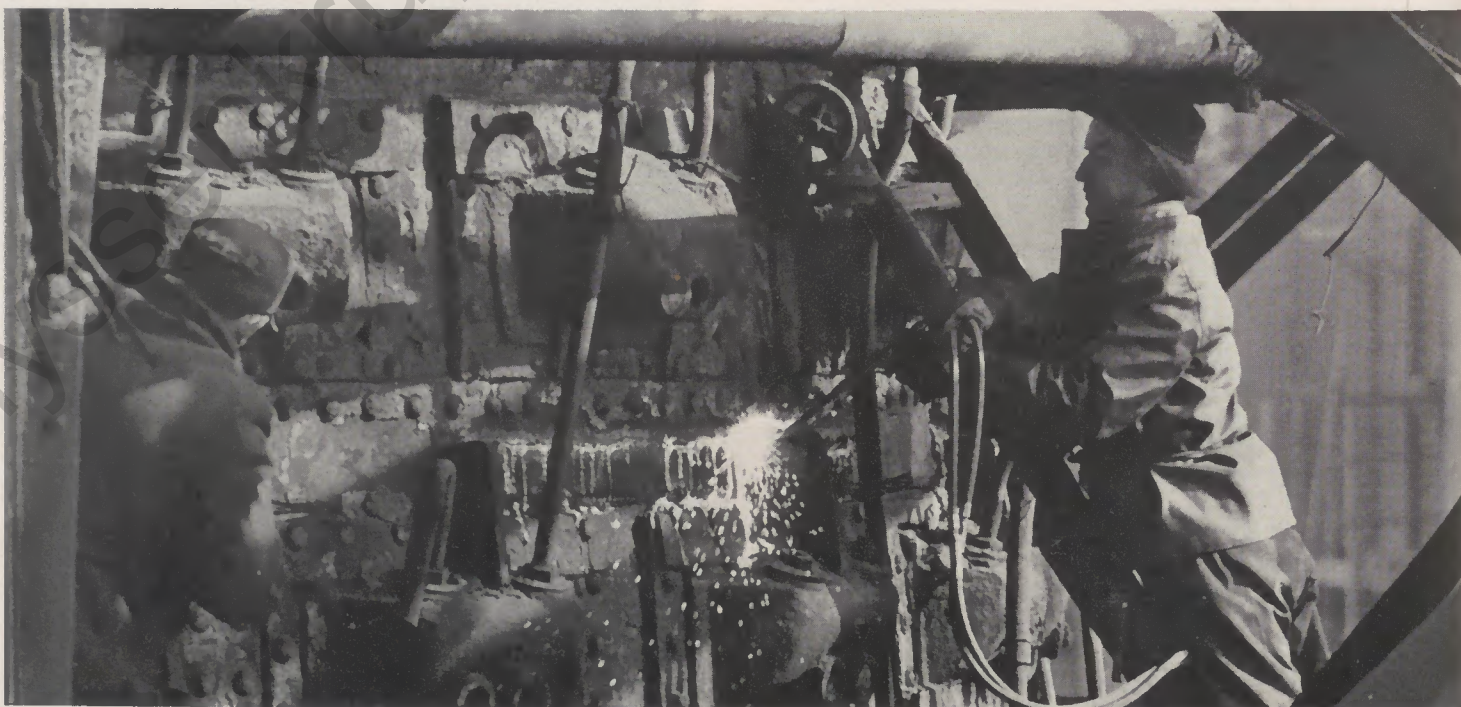
Demontage 1960: Kaum noch als Hochofen identifizierbar ist das Stahlgerüst, das noch immer den Ofenschacht umschließt; (o.); doch schon rücken die Schneidbrenner auch dem Panzer zu Leibe (u.). Bei der Demontage eines Winderhitzers (o. r.) erkennt man den aus 60 000 Gittersteinen bestehenden Besatz
