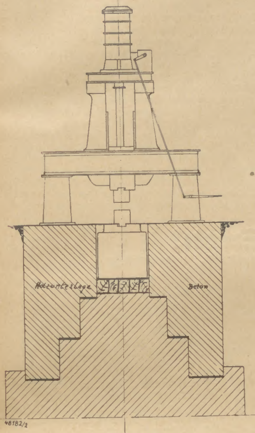
Abb. 4: Dampfhammer mit Fundament
