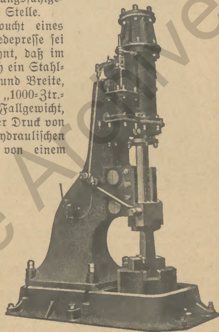
Abb. 6: Einständerhammer
