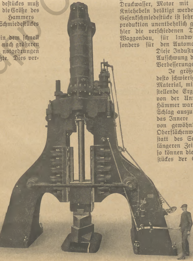
Abb. 5: Stahlhämmer von 7500 Kilogramm Fallgewicht
