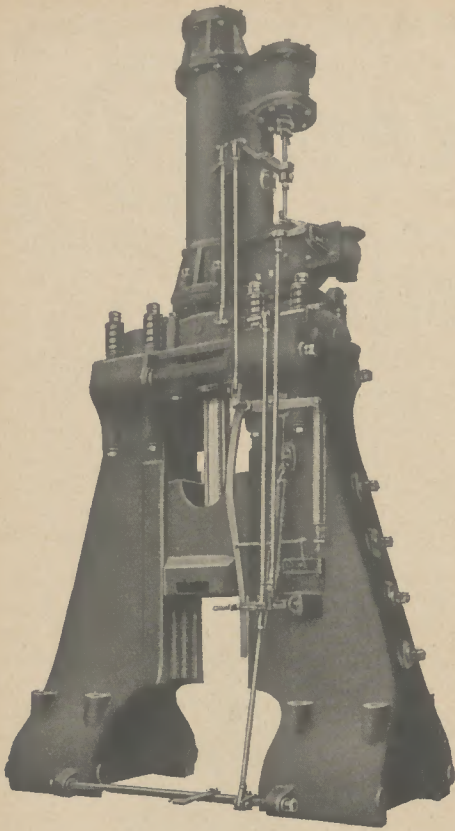
Abb. 7: Spezialgeßelhammer System „Eric“ zum Ausschlagen von Massenartikeln
