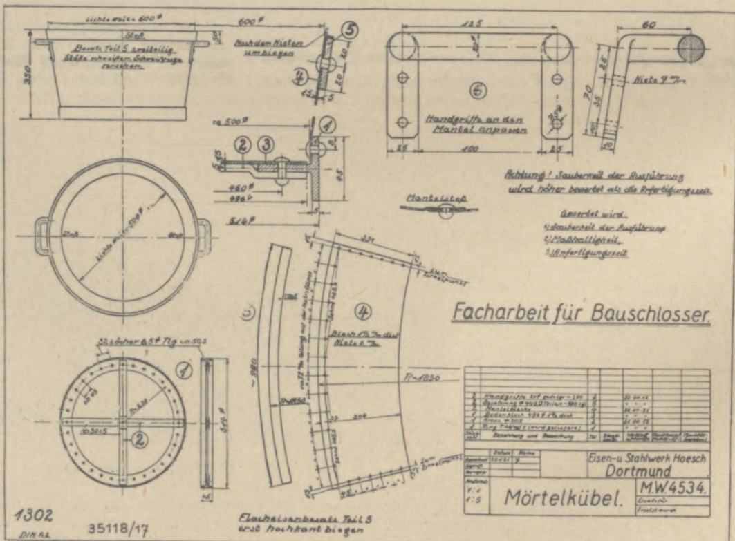
Bild 3: Facharbeit für Bauschlossler: Mörtelkübel, Aufgabe
