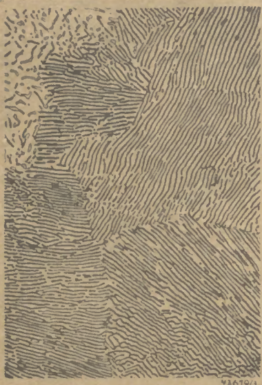
Abb. 4: Gefüge des geglühten Stahles, Perlit (500 X)
