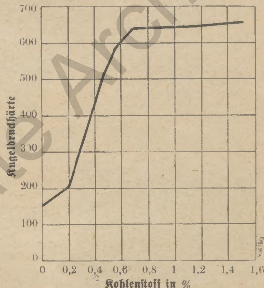
Abb. 3: Änderung der Härte des abgeschreckten Stahles mit steigendem Kohlenstoffgehalt
