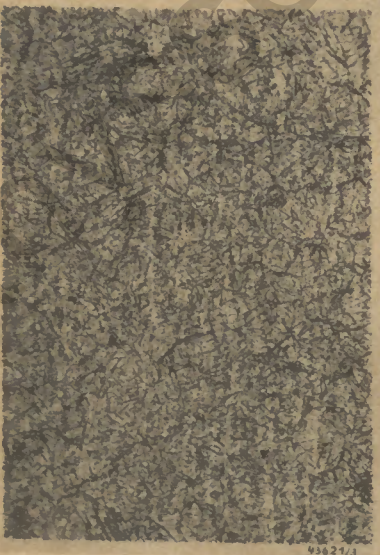
Abb. 6: Gefüge des vollkommen gehärteten Stahles, Martensit (500 X)
