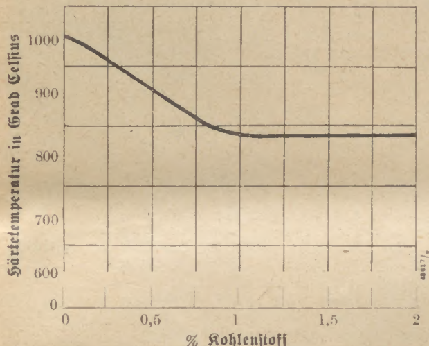
Abb. 2: Änderung der Härtetemperatur mit dem Kohlenstoffgehalt
