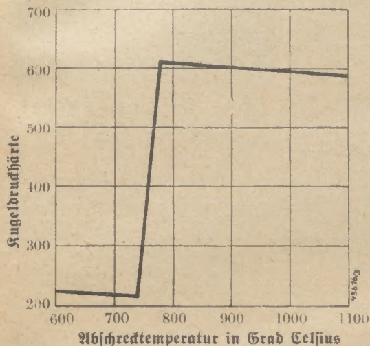
Abb. 1: Härteänderungen eines Stahles mit 1% Kohlenstoff durch Abschrecken von verschiedenen Temperaturen
