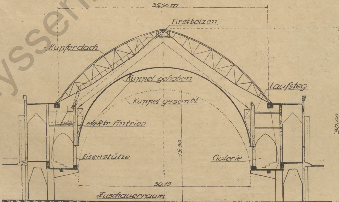
Querschnitt durch das Planetarium.
