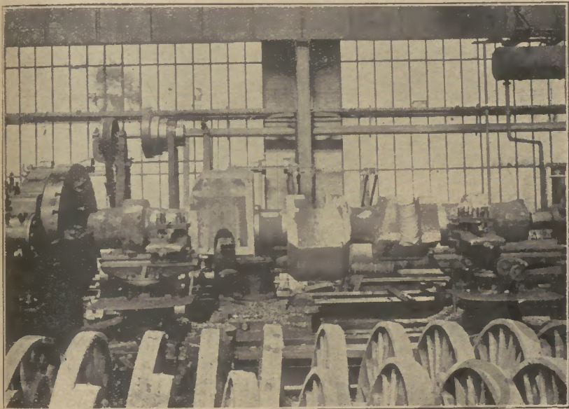
Welle auf der Schruppbank.
