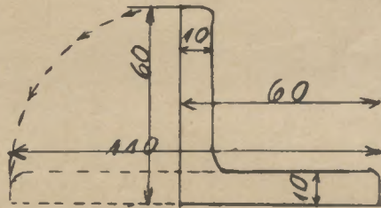
Gleichschenkliges Winkelisen.
