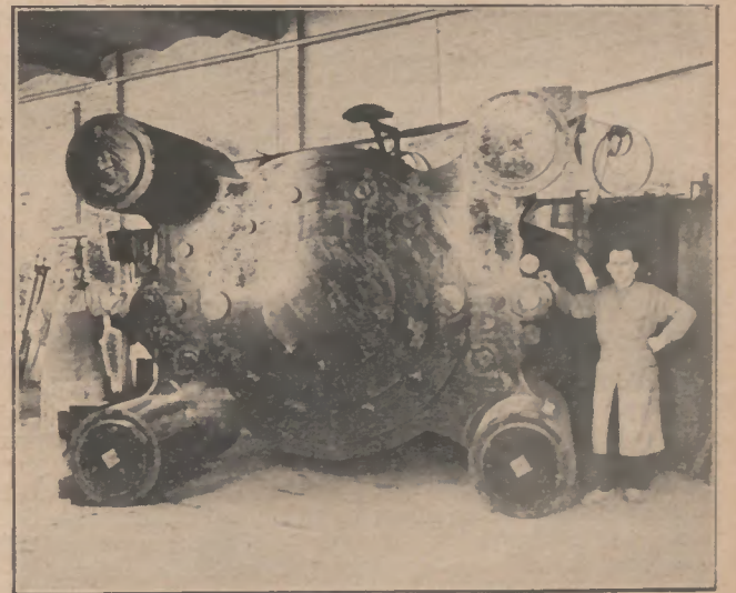
Bewegl. Querkopf zur 3000 Tonnen-Pressen im Presswerk.
