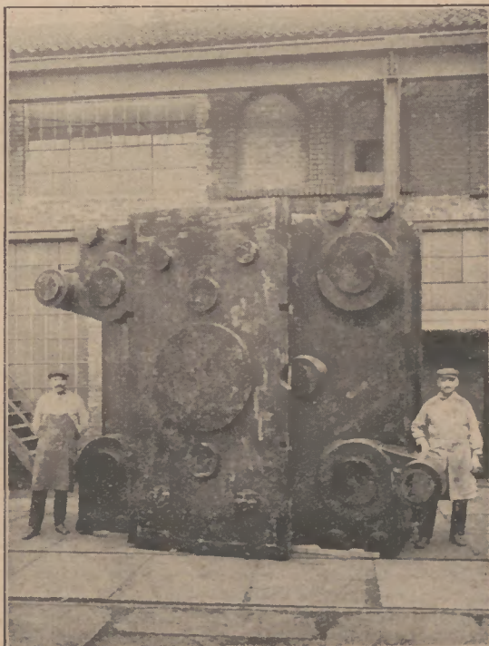
Weitere Arbeiten der Modellschreinerei der Mech. Werkst. der Dortm. Union: Presszylindermodell für die 3000 Tonnen-Pressen der Presswerke.
