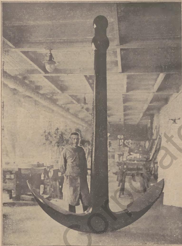
3000 Kilogr. Union-Stodantermodell für die Stahlformgießerei, hergestellt von der Modellschreinerei der Mechanischen Werkstatt der Dortmunder Union.
