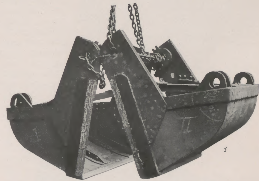
Abb. 57: Instandgesetzter Greifer, auf dessen Schneidenflächen Manganelektroden aufgeschweißt sind
