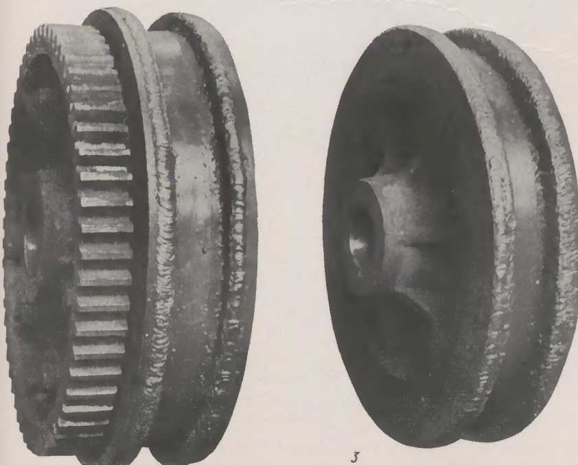
Abb. 55: Laufräder mit elektrisch aufgeschweißten Spurkränzen
