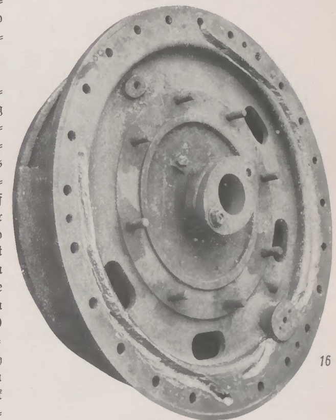
Abb. 68: Gußeiserner Pumpendeckel zum Schweißen vorbereitet; Risse ausgekreuzt
