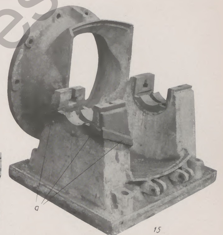
Abb. 67: Gußeisernes Kurbelgehäuse und Lagerdeckel nach Abb. 66, durch elektrischer Warmschweißung instand gesetzt. Bruchstellen a verstärkt
