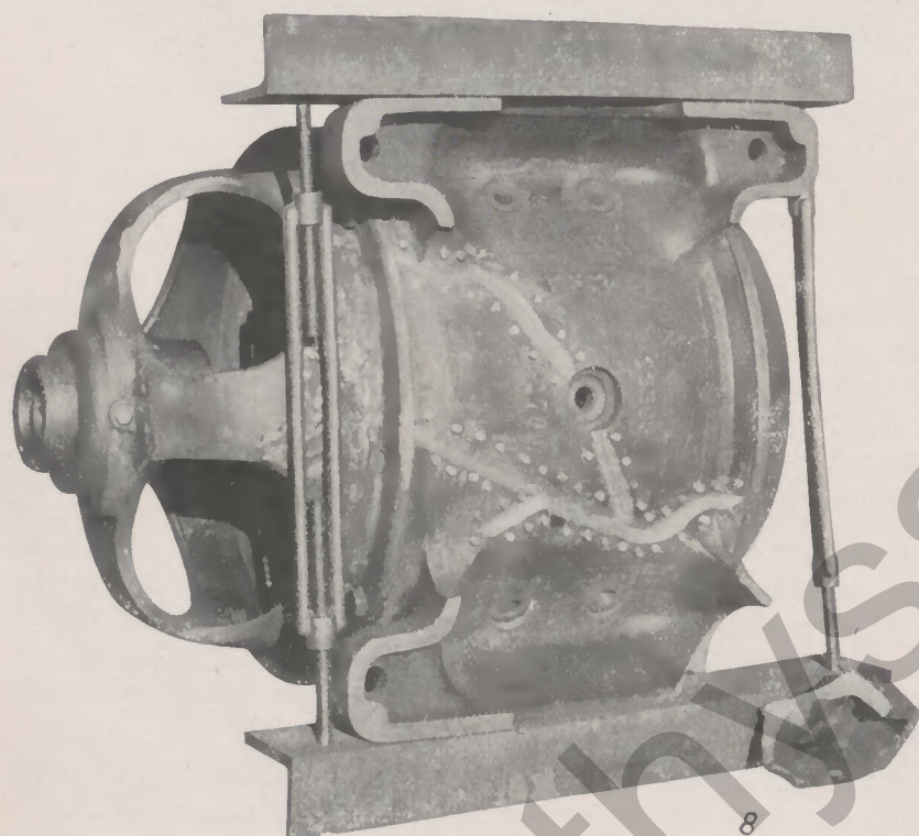
Abb. 60: Gesprungenes, gußeisernes Motorgehäuse, zur Kaltschweißung vorbereitet. Die Risse sind ausgekreuzt, die Schraubstifte eingesetzt.
