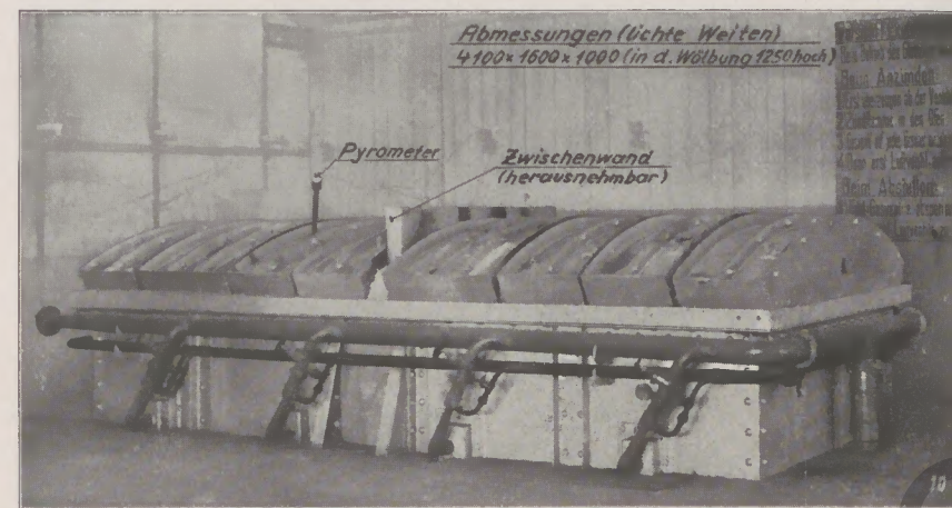
Abb. 62: Schweiß- und Glühofen
