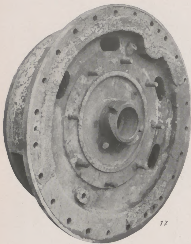
Abb. 69: Gußeiserner hohlwandiger Pumpendeckel, wie Abb. 68, warmgeschweißt und spannungsfrei geglättet
