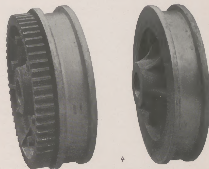
Abb. 56: Geschweißte Laufräder nach Abb. 55, fertig bearbeitet
