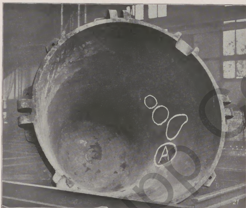
Abb. 73: Halbwarmgeschweißte Fliesen in einer durchgebrannten gußeisernen Hochofenschladenpfanne. A ist alter Fliesen
