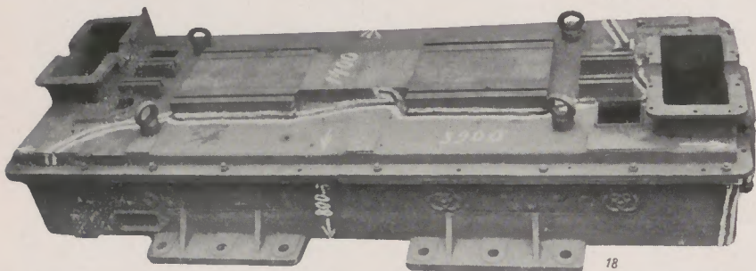
Abb. 70: Traversen zur Zentralanstellung einer Plattierungswalze im Blechwalzwerk III. Risse ausgekreuzt. Gewicht 5600 Kilogramm
