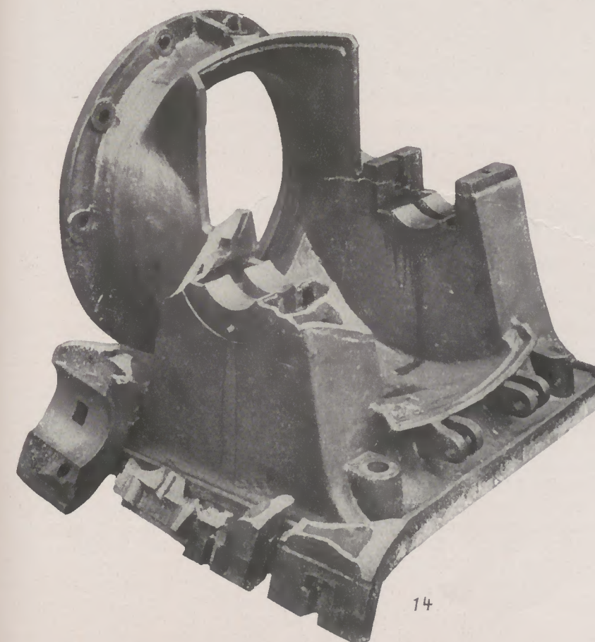
Abb. 66: Gußeisernes Kompressor-Kurbelgehäuse mit gebrochener Lagerstelle und Lagerdeckel
