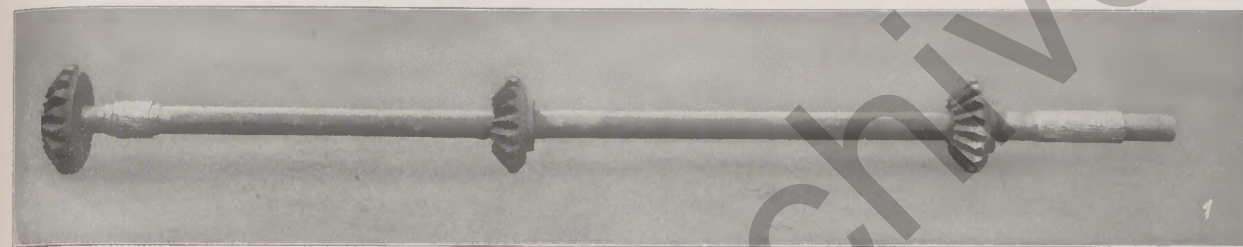
Abb. 53: Auftraggeschweißte Rollgangswelle
