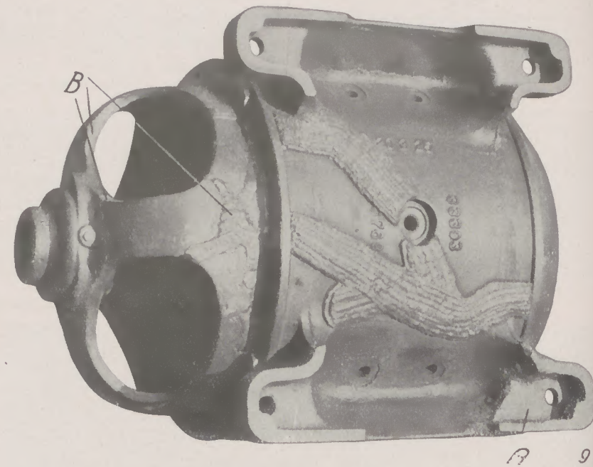
Abb. 61: Gußeisernes Motorgehäuse nach Abb. 60. Kaltgeschweißt. Fuß A und Lauffstellen B im Lagerschild sind halbwarm autogen geschweißt.
