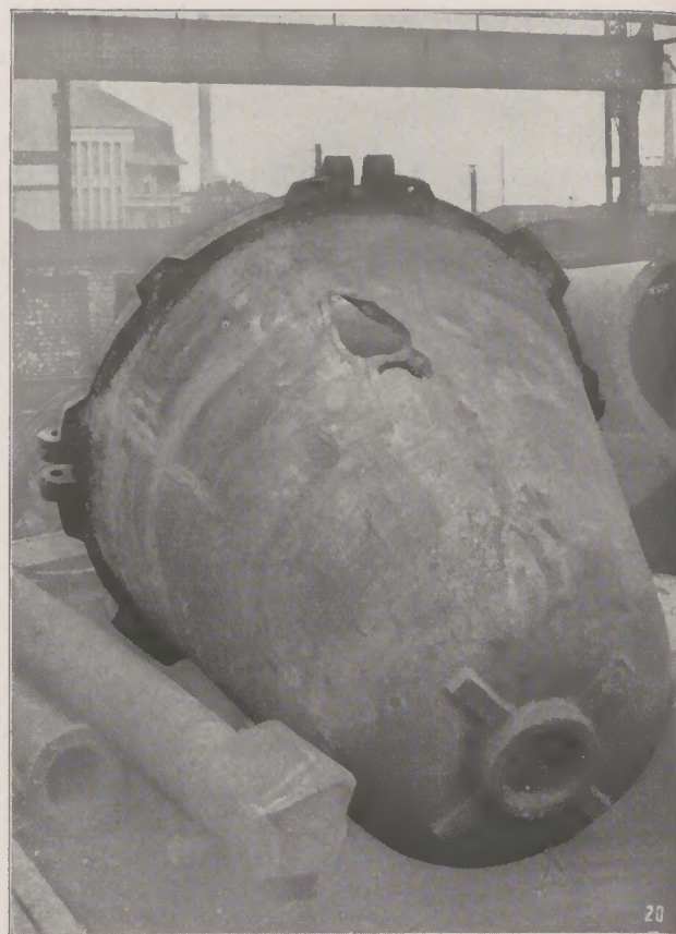
Abb. 72: Durchgebrannte gußeiserne Hochofenschladenpfanne
