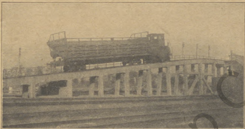
Kokslöschwagen.
