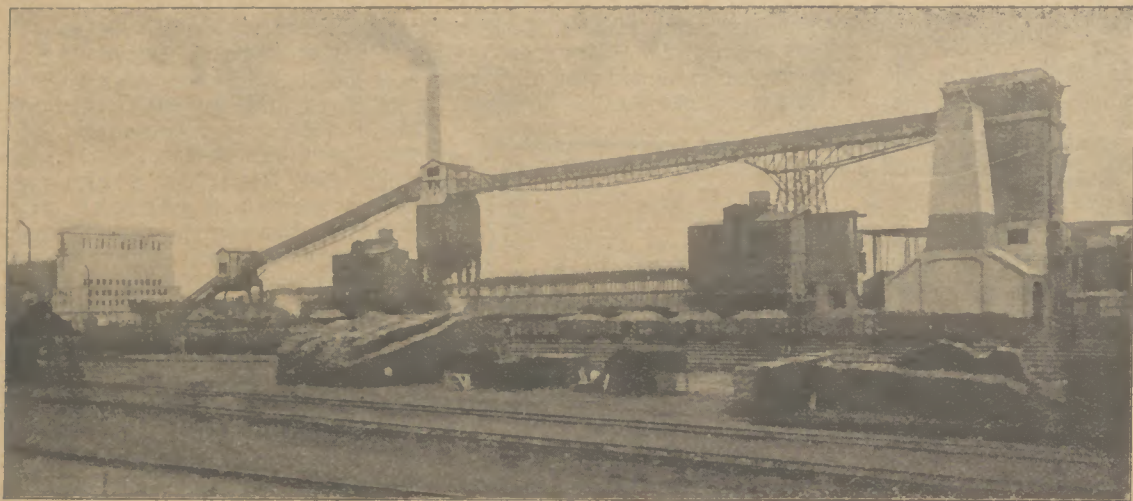
Blick über Holzplatz und Sechenbahnhoi auf Koker- und Kokslozentransportanlage der Gewerkschaft Auguste Viktoria.
