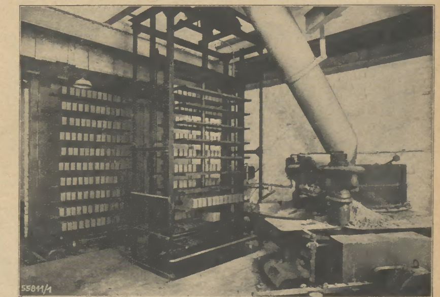
Drehzylinder mit Hubgerüst
