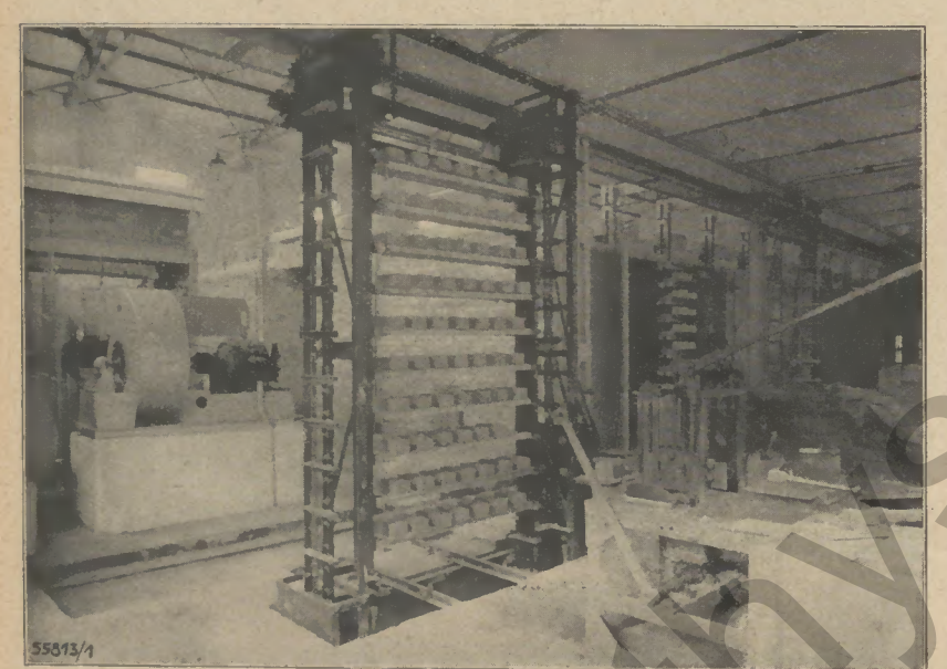
Silika-Trockenanlage, vorn: Handpresse mit Abseggerüst
