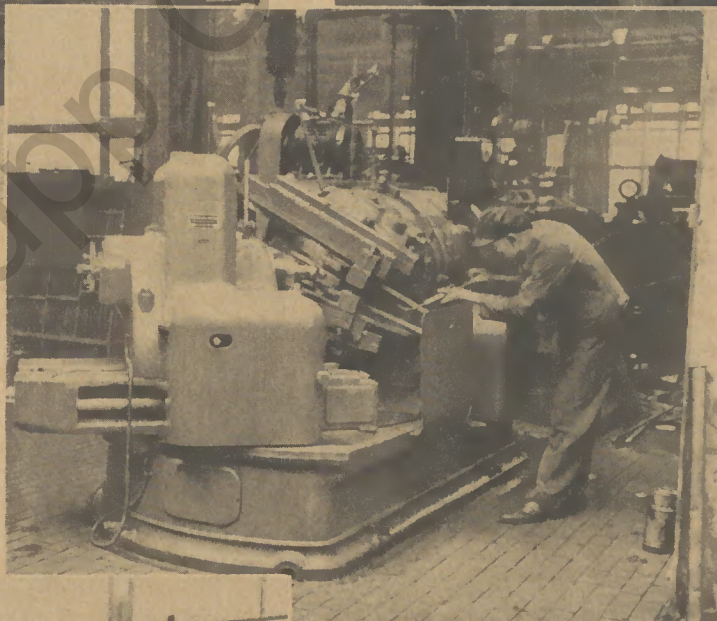
Bild rechts nebenstehend: Ein schöner Arbeitsplatz (Kegelradhobelapparat in der Zahnradfräselei)
