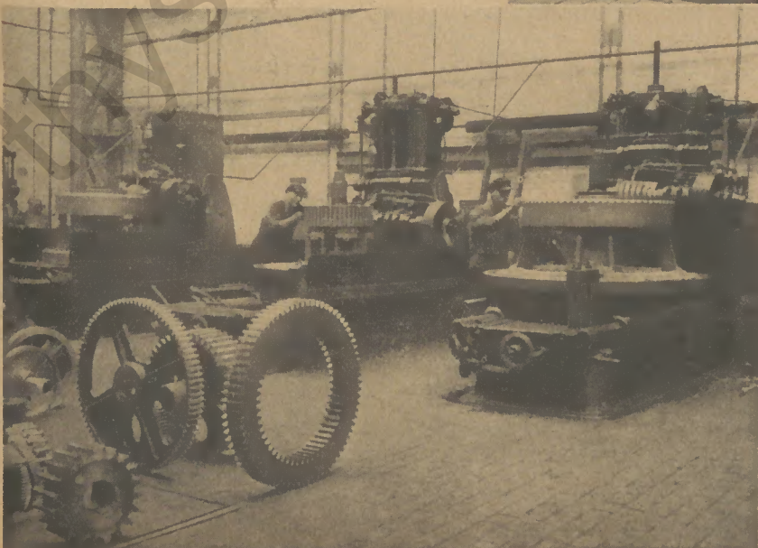
Bild rechts nebenstehend: Ein schöner Arbeitsplatz (Kegelradhobelapparat in der Zahnradfräselei)
