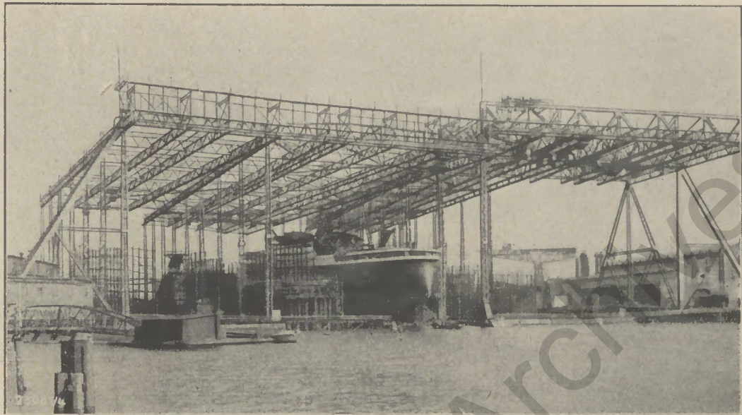
Die große Helgenanlage vor dem Werfthafen Blohm & Voß
