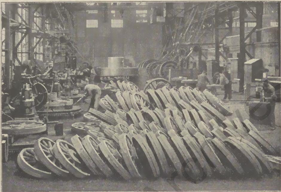
Locomotiv-Radsterne in der Stahlgußhütte
