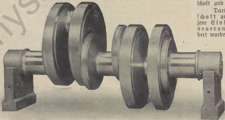
Zweihübrige Pol.-Kropfschse aus Nickelstahl für den Treibradsatz einer Schnellzuglokomotive
