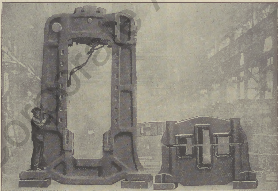
Stahlgußwalzenständer von 21 To. Stückgewicht und Kammwalzenengerüst mit Deckel von ca. 13,5 To. Gewicht
