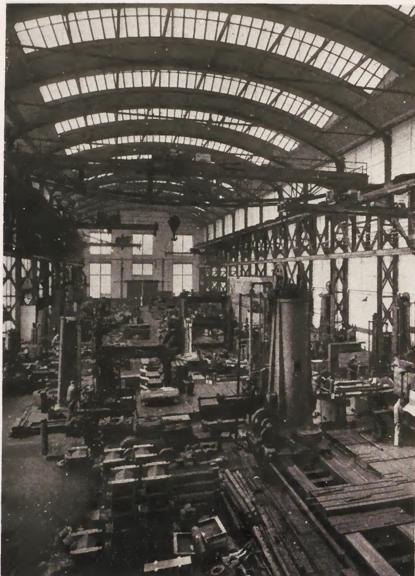
Bearbeitungswerkstatt im Eisenwerk Wanheim
