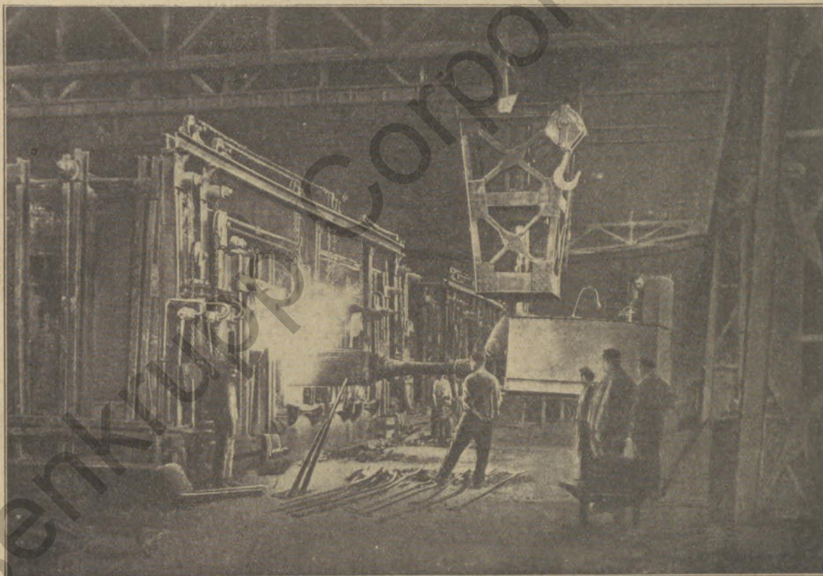
Im Siemens-Martin-Stahlwerk.
