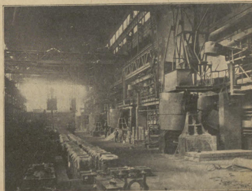
Gießhalle.
