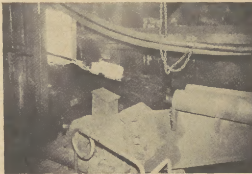
Schnell einen Blick auf die dem Ofenmann gegenüberliegende Ziehlüre. Da wird gerade ein Block mit dem Greifer gegriffen und auf einen Rollgang gelegt, der ihn zur Entzunderung weiterbefördert.
