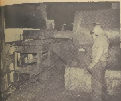
Anton Lecht überzeugt sich durch einen Blick in den Ofen, ob die Blöcke von der Einstoßseite her, ob die Blöckchen die vorgeschriebene Bahn laufen.
