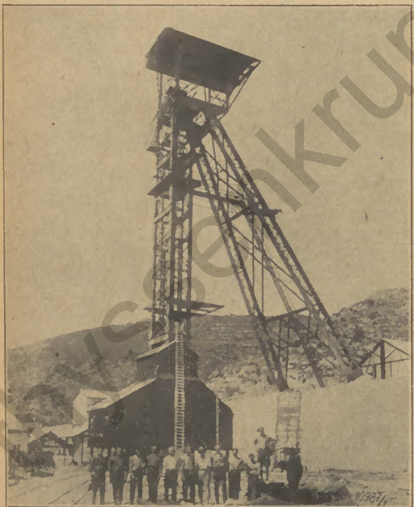
Das von der Dortmunder Union in Spanien für den Kalischacht Niéves erbaute Fördergerüst
