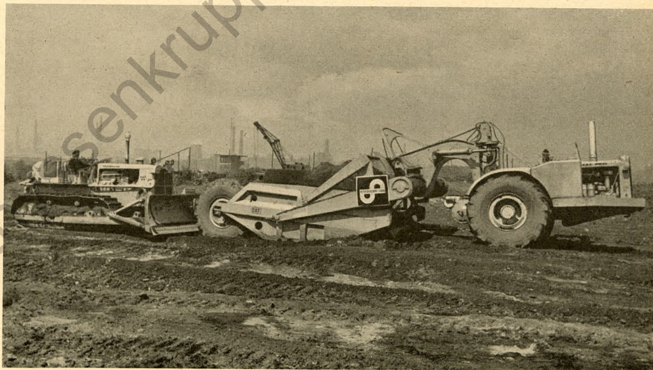
Abb. 3 Die hintenfahrende Raupe schiebt den Scraper
