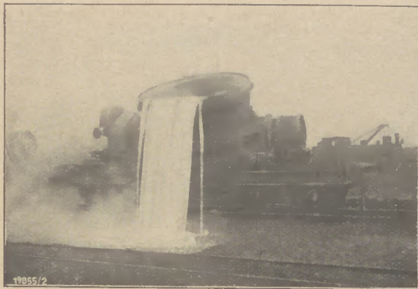
Bild 1: Eingießen der flüssigen Schlacke in Betten
