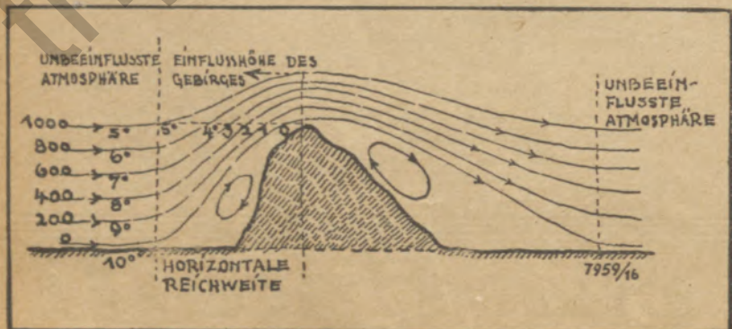
Luftströmungen an Bergabhängen
