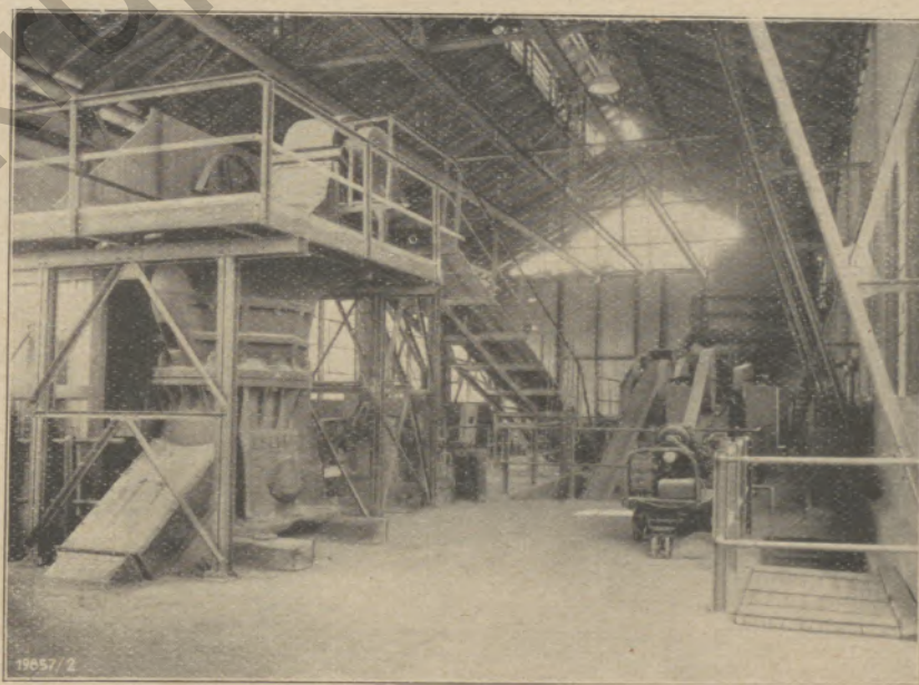
Bild 3: Innenansicht der Brecheranlage
