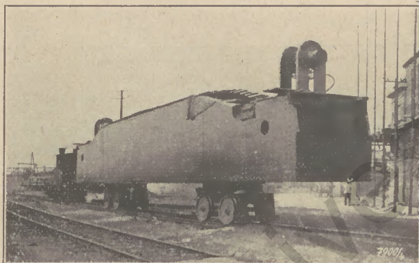
Transport der Ballastkästen für die Königinbrücke in Rotterdam
