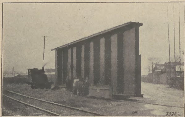
Drehschmelzwagen mit Flutbrückenträger für die Düsseldorf-Brücke
