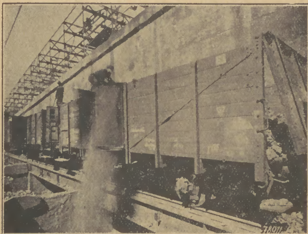
Das unsichere Kotswagenöffnen vom beladenen Kotswagen
