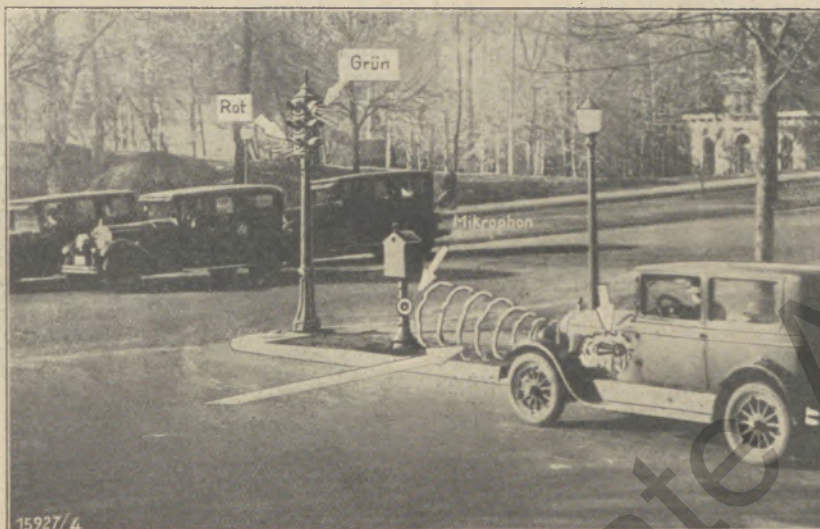
Der moderne Kraftwagen als akustischer Signalauslöser Die von der Hupe kommenden Schallwellen treffen auf das Mikrophon und betätigen die Lampen
