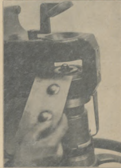
Abb. 4: Prüfergerät zur Feststellung der Tiefziehfähigkeit von Blechen nach Erichsen
