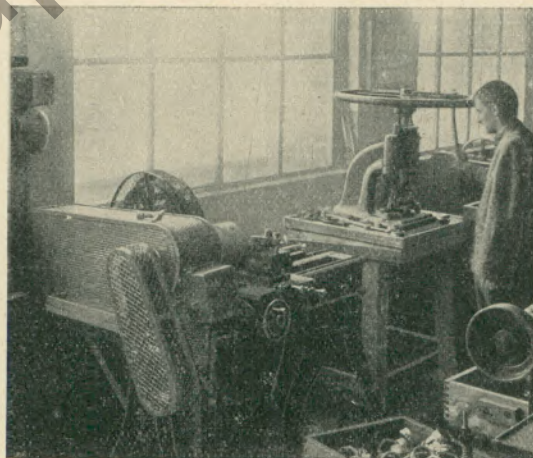
Bedienung einer Handhebelpresse und halbautomatischen Drehbank zugleich. Das Arbeitsstück wird in das Drehfutter eingespannt und die Maschine eingerichtet. In der Zwischenzeit wird die Handhebelpresse bedient, bis an der Drehbank das Werkstück fertig ist, was durch eine elektrische Klingel gemeldet wird. Kriegsblinder mit gelähmtem linken Arm.
