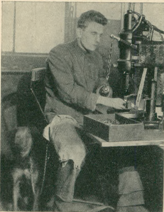
Abb. links: Sentrechte Gewindeschneidmaschine für einarmigen Kriegsblinden mit verkrüppelter rechter Hand eingerichtet. Mit den Stummeln der rechten Hand werden die Teile aus dem Kasten genommen, auf dem rechten Knie in die richtige Lage gebracht und dann in die an der Maschine besonders befestigte Haltevorrichtung eingeschoben. Mit der am linken Unterarm befestigten Prothese wird mittels einer damit verbundenen Gliederkette der Handhebel heruntergezogen. Ein automatischer Auswerfer befördert die Teile in einen Kasten.
