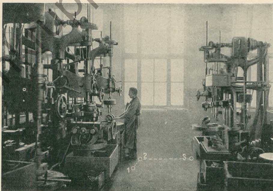
Drei große Halbautomatische Bohrmaschinen werden zugleich von einem Blinden bedient. Gußkörper einlegen und bohren (8 Löcher).
