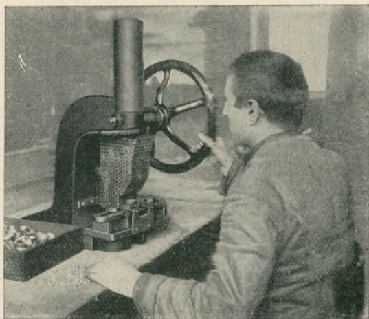
Nietarbeiten werden an der Kornpresse ausgeführt. Um Verletzungen zu verhindern, ist ein bewegliches Schutzgitter angebracht, welches bei Betätigung des Handrades sich vorwärtsbewegt und die Hand freiräumt.
