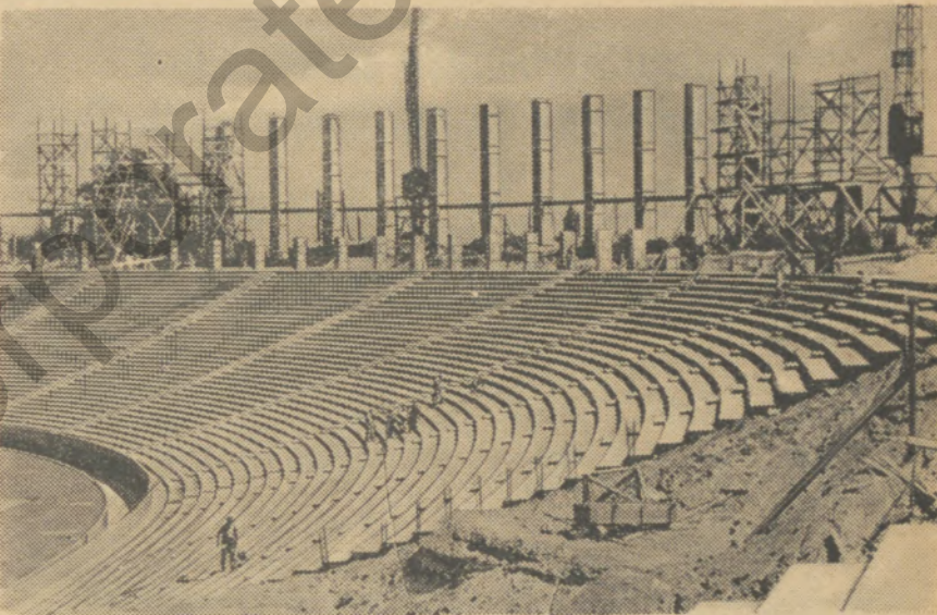
Baueisenbau im Olympia-Stadion
