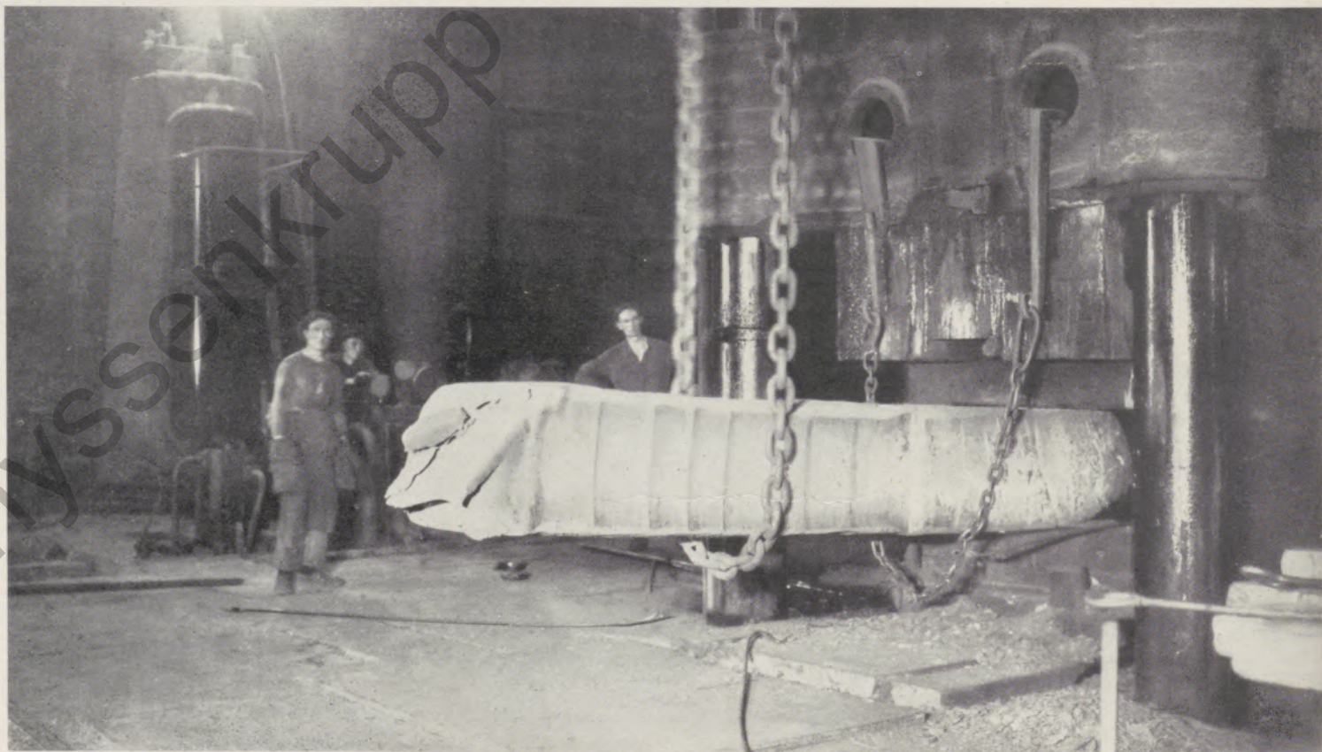
Bild 4: Schmiedepresse; Schmieden eines Stahlblockes für Kaltwalzen
