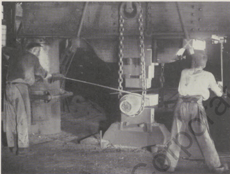
Bild 3: Dampfhammer mit 40 Ztr. Bärgeviert für das Anschmieden von Stahlblöcken
