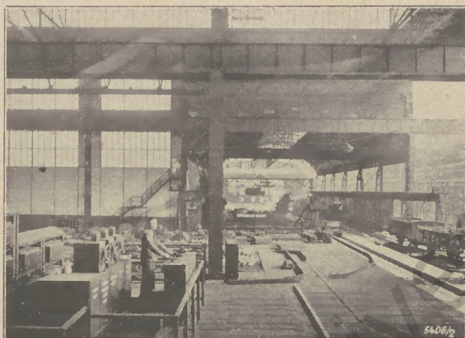
Bild 7: Kollgänge, Warmjagen und Warmlager
