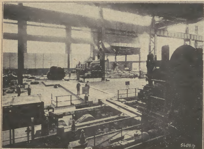
Bild 6: Quertransport des vorgewalzten Stabes
