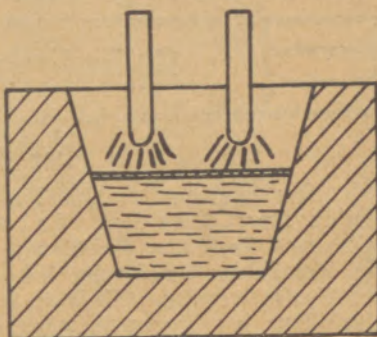
Figur 1: Lichtbogenheizung a) Die direkte Heizung (Héroult-Ofen) die Schmelzmasse ist der direkten Wärmewirkung ausgesetzt.
