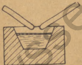
Fig. 3: Die indirekte Heizung, sog. Strahlungsheizung. Hier brennt der Lichtbogen außerhalb und strahlt lediglich seine Wärme auf die Schmelzmasse.
