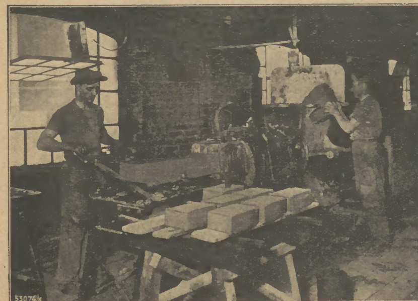
Strangpresse — Ein Pfannenstein wird „vorgezogen“
