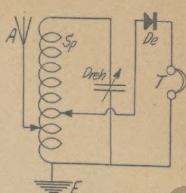
Abb. 4: Schema des beschriebenen Empfängers.
