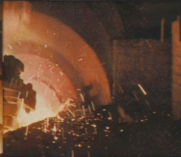
▲ Der Abstich läuft. Weißgelb strömt das Eisen durch die Abstichrinne. Die erste Pfanne unter der Ofenbühne ist gefüllt; nun dämmen die Schmelzer die Rinne ab und öffnen dem Eisen einen neuen Weg
