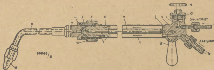
Bild 4: Schweißbrenner
